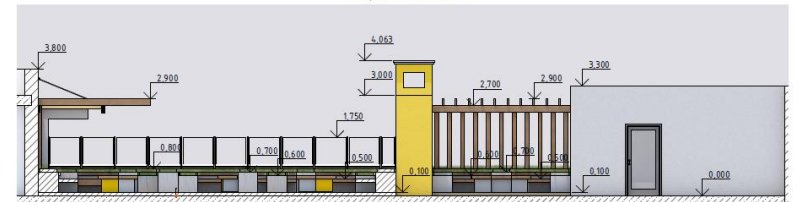
Розріз 2 - 2, м 1:50
