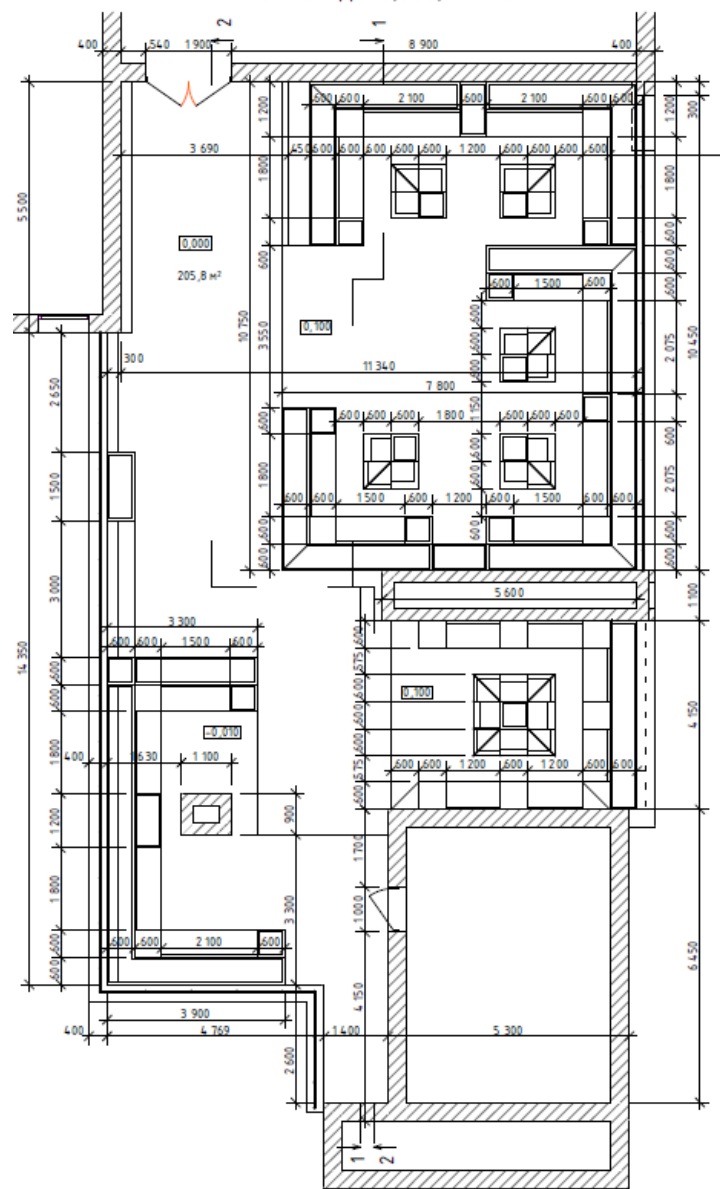
План на відм. 0,000, м 1:70
