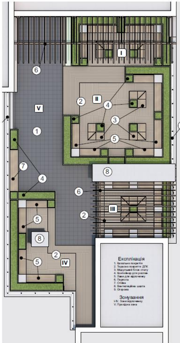
Генплан, м 1:50
