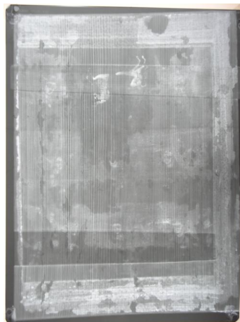
Рентгенограма
