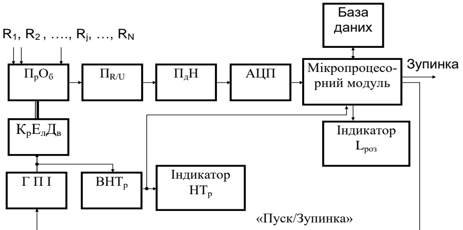
Рис. 1. Схема роботи системи з моніторингу розриву тросів вантового канату
